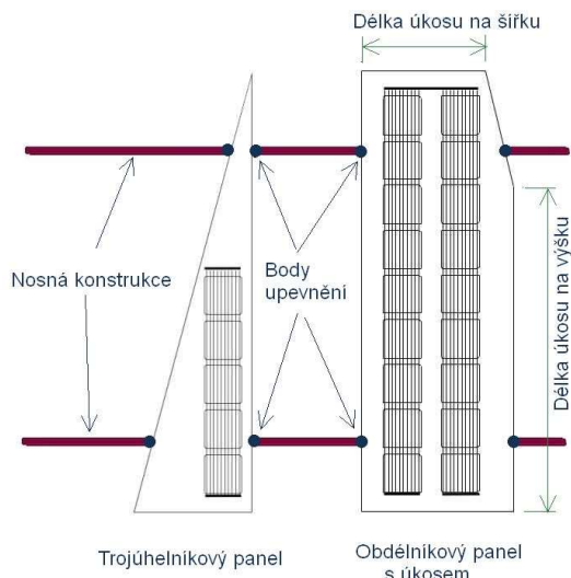
Obrázek č. 2 - Technický výkres panelu řady 400
