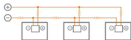
Paralelní zapojení
