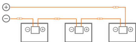
Sériové zapojení
