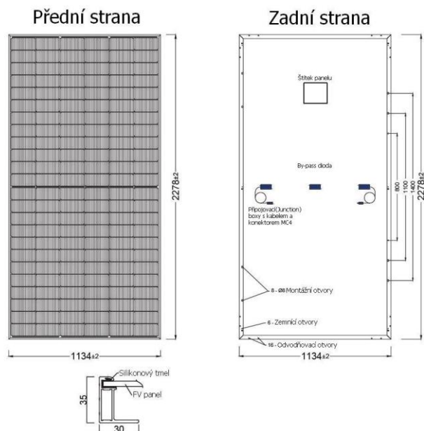
Obrázek č. 2 - Technický výkres panelu řady FD590
