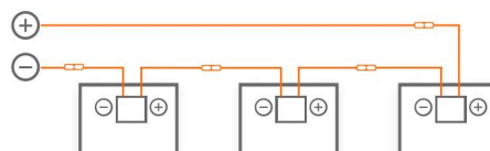
Sériové zapojení
