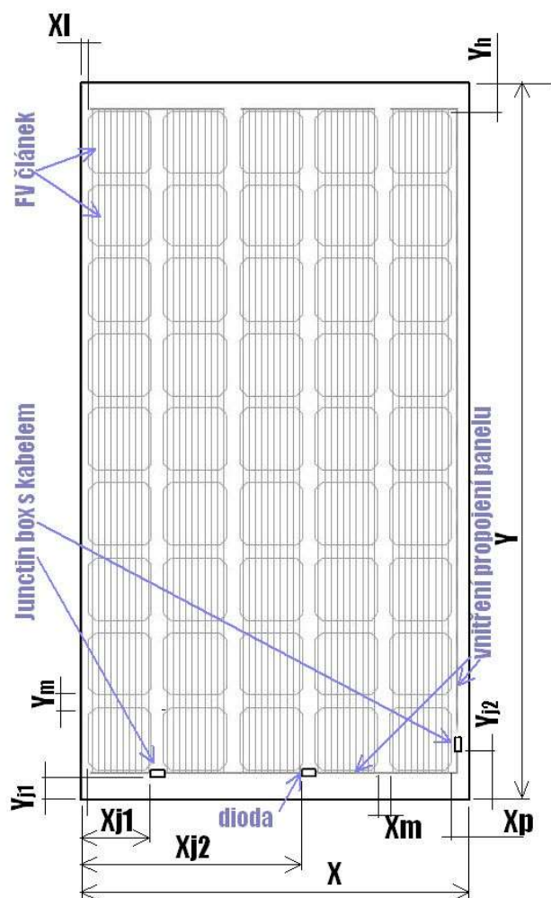
Obrázek č. 2 – Obecný výkres transparentních panelů
